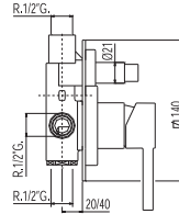
Monomando empotrar baño-ducha
